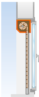
Sous linteau avec enroulement extérieur
