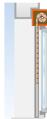
Intégré à la fenêtre et visible de l'intérieur de la pièce
