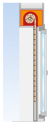
Intégré dans la maçonnerie
