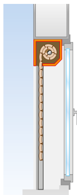
Sous linteau avec enroulement intérieur
